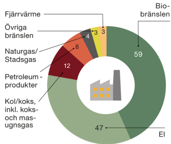
Industrisektorns slutliga energianvändning 2020, TWh
